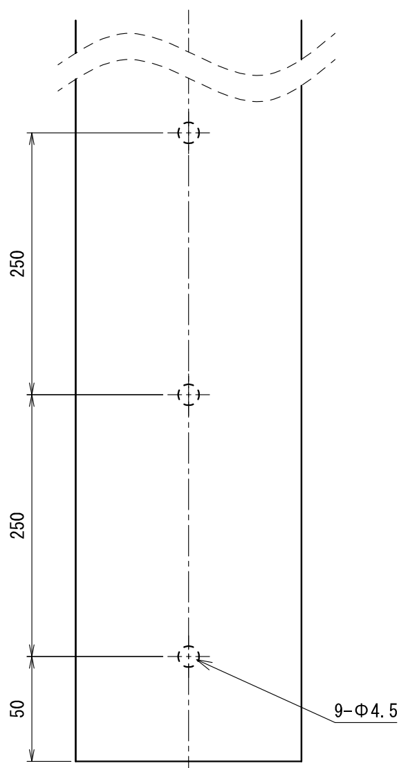
ビス取付穴ピッチ
